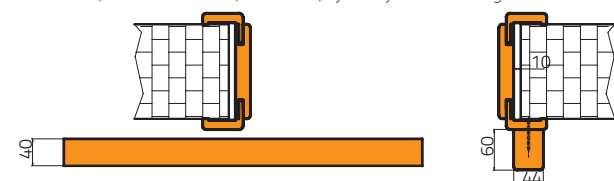
Návkres 1. Horizontálny rez posuvného nastenného systému - dorazova lišta ľavá
