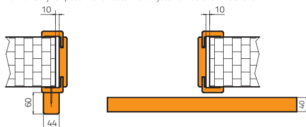
Návkres 2. Horizontálny rez posuvného nastenného systému - dorazova lišta pravá
