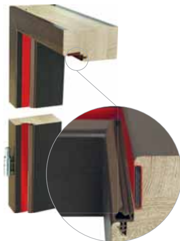
klešajúce tesnenie naspodu krídla (verzia 2)
