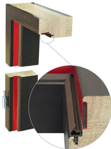
klesajúce tesnenie nasponu krídla (verzia 2)
